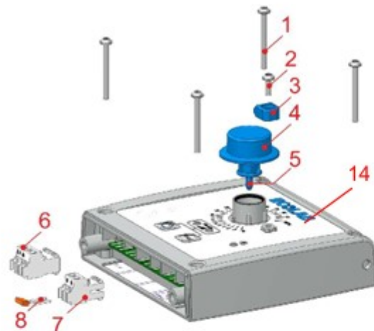
Řídicí jednotka
